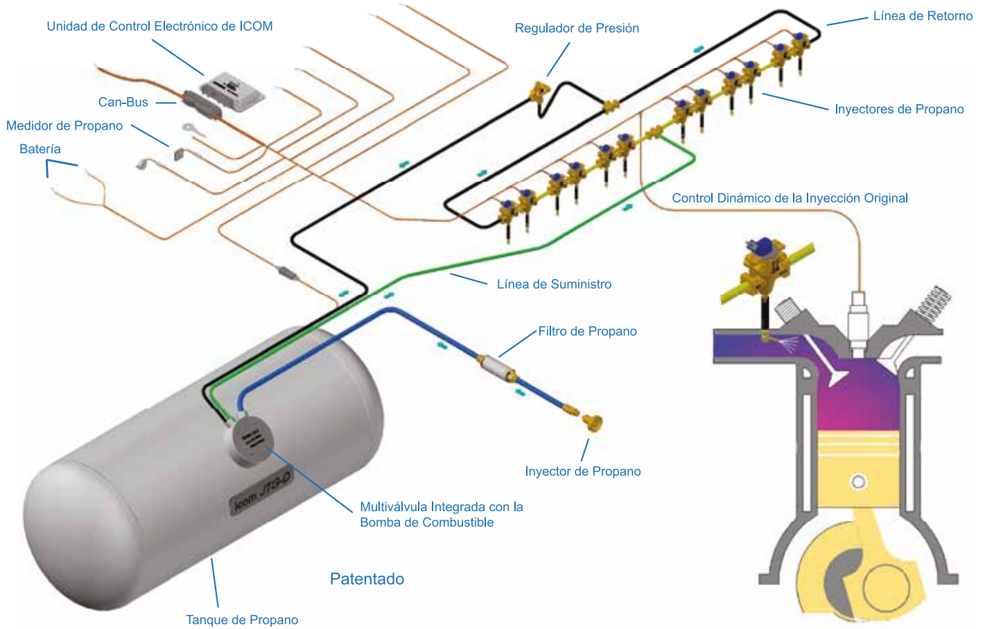
JTG-Dynamic Reducción de Emisiones
