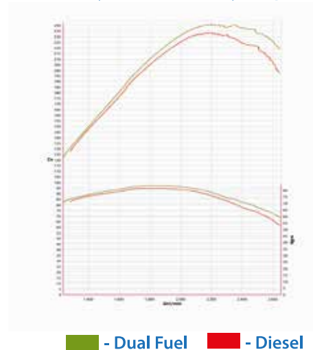
JTG-Dynamic Potencia y Torque
